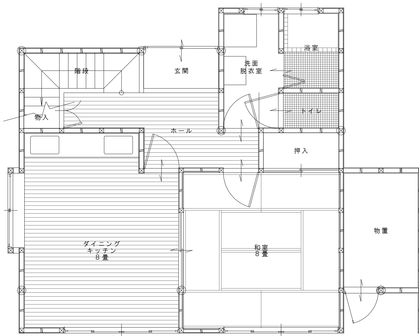
1 階平面図
