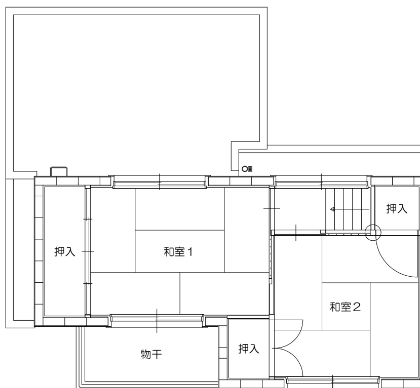
2階平面図
